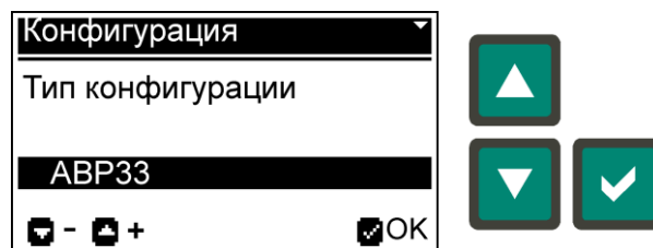
Рис. 5.18. Меню «Конфигурация»
