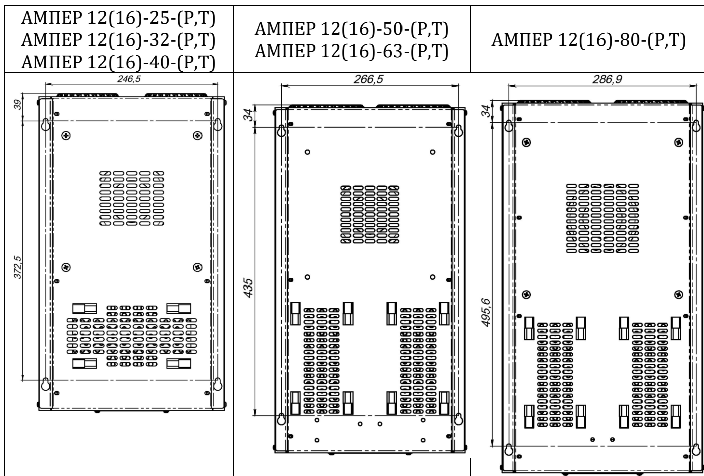
Рисунок 4. Установчі розміри стабілізаторів
