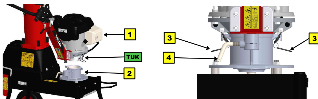
Obr. 3: Připojení pohonné jednotky
