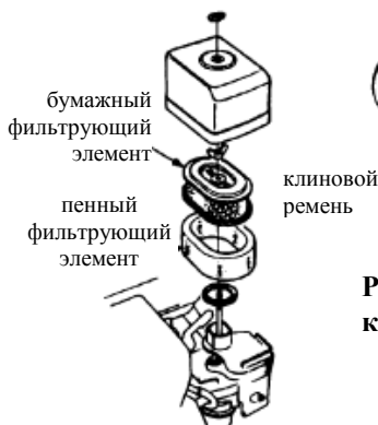
Рисунок 1. Воздушный фильтр
