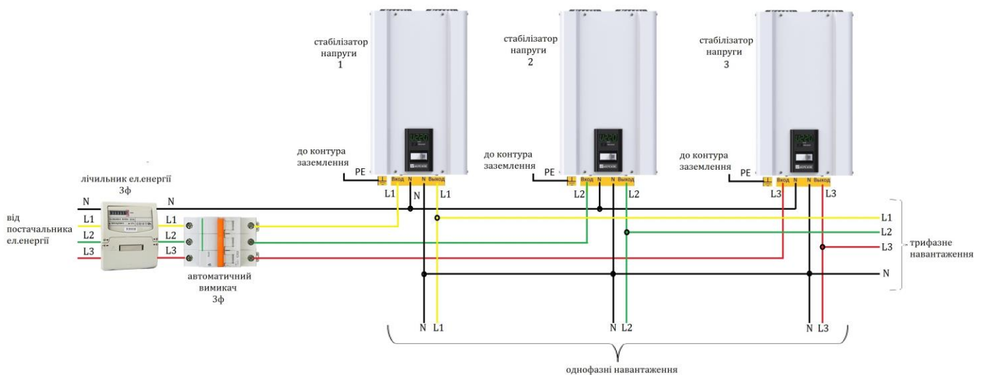
Рисунок 7. Схема підключення стабілізатора до трифазної мережі
