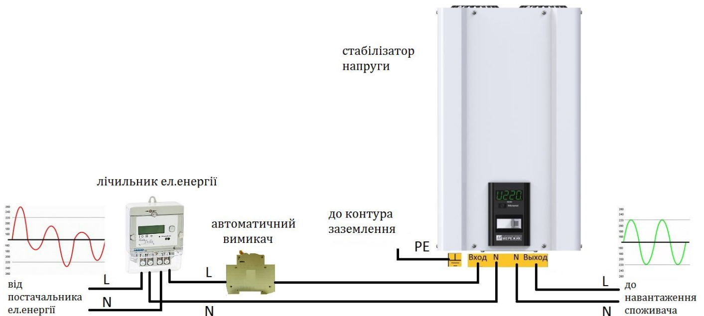
Рисунок 6. Схема підключення стабілізатора до однофазної мережі
