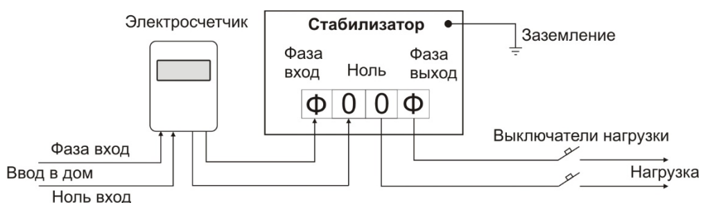
Рис.6 – Схема підключення стабілізатора до однофазної мережі
